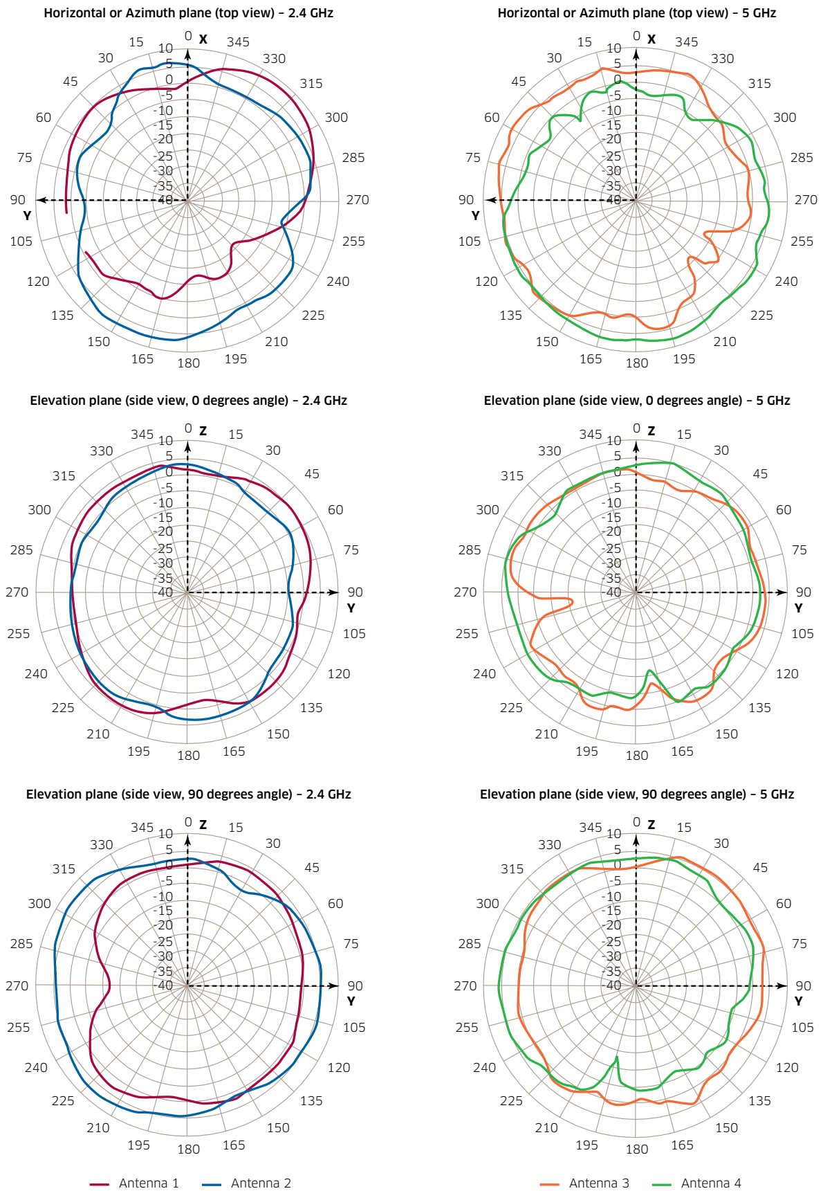
Abbildung 1: OmniAccess AP1101-Antennenmuster
